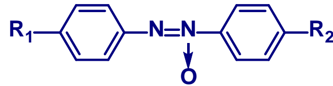
Азоксибензолы
