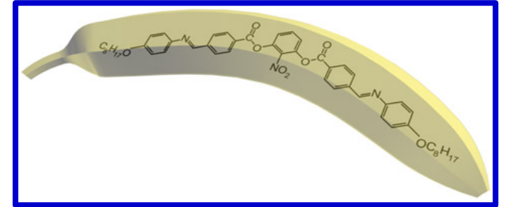
бананоподобные молекулы
