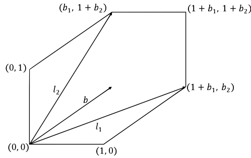
Рис. 1. Вытягивание единичного квадрата
