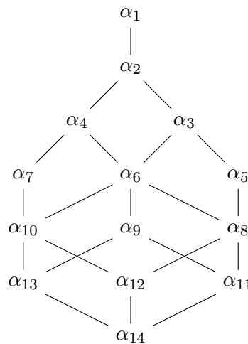
Рис. 2. Диаграмма Хассе множества S_{T(4,2)} .
