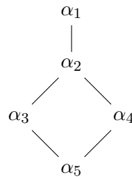
Рис. 1. Диаграмма Хассе множества S_{T(4,1)} .
